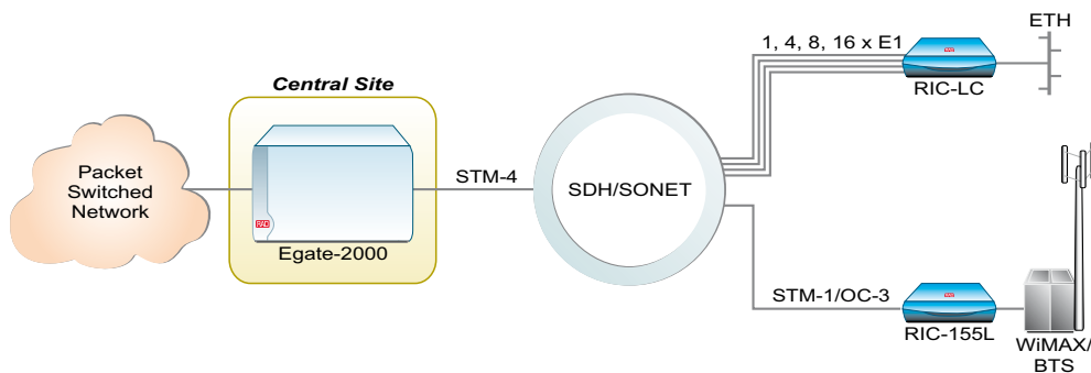
Транспорт трафика Ethernet через PDH и SDH
