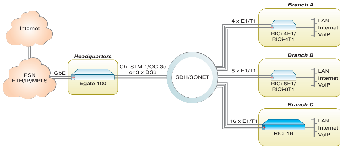
Дифференцированные бизнес-услуги Ethernet по связанным линиям PDH
