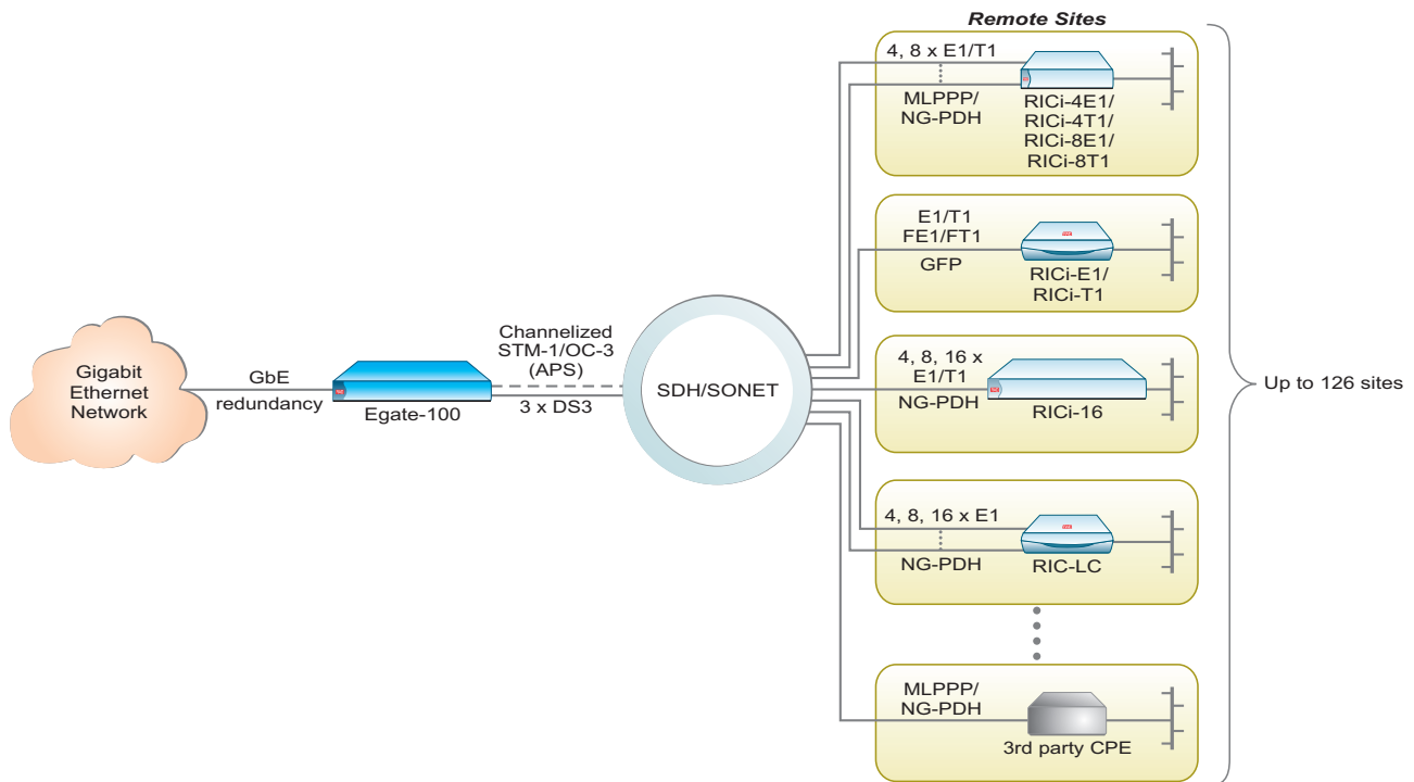
Объединение трафика Ethernet по структурированным каналам STM-1/OC-3 или 3 x DS3
