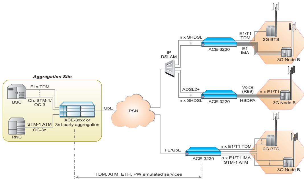
Совмещение базовых станций 2G -3G и доступ к PSN
