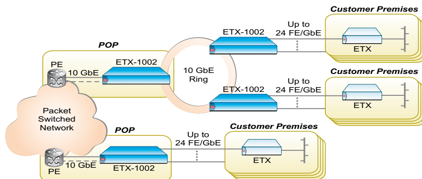
Высокоскоростной транспорт и агрегация услуг по кольцу 10 GbE
