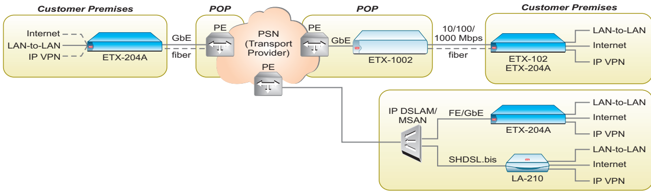
Демаркация услуг Ethernet в пакетных сетях с управлением от площадки пользователя
