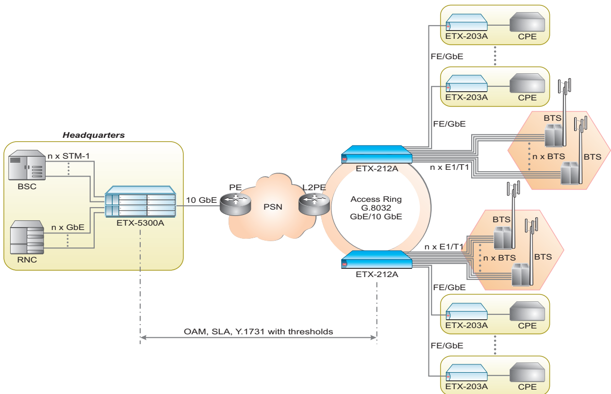
Демаркация услуг Ethernet в пакетных сетях и устойчивый доступ по кольцу
