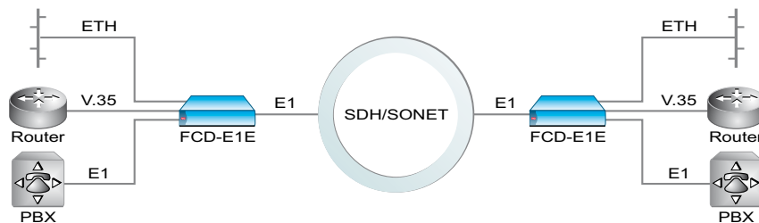
Передача данных по E1 между двумя точками
