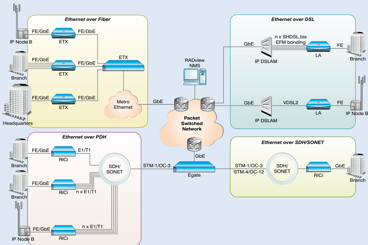
Операторский Ethernet-доступ по любой транспортной сети
