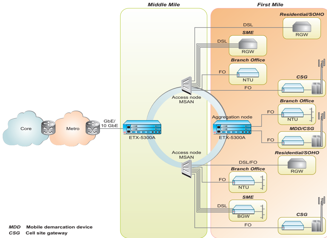
ETX-5300A агрегирует трафик на «первой миле» и «средней миле»
