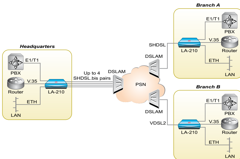
Передача традиционных услуг и Ethernet по инфраструктуре SHDSL.bis и VDSL2
