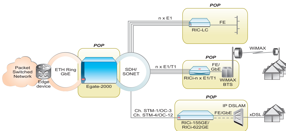
Услуги Ethernet и транспорт трафика через PDH/SDH/SONET
