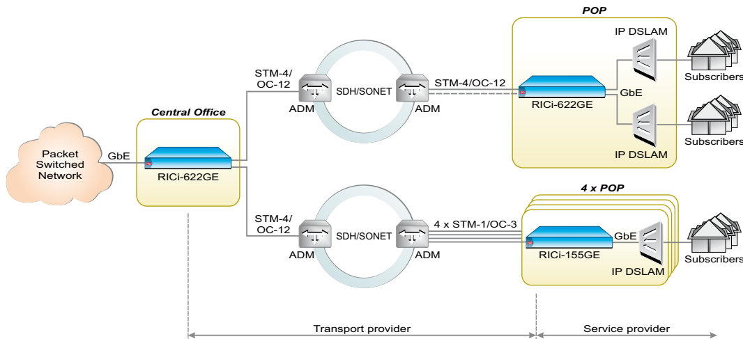
Подключение IP DSLAM через сетевые каналы STM-4/OC-12
