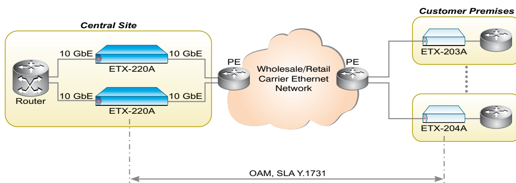
Доступ по 10 Gigabit Ethernet
