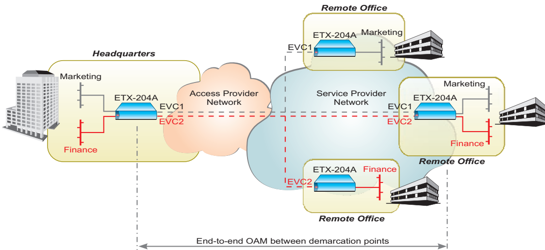
Передача услуг Carrier Ethernet по различным сетям
