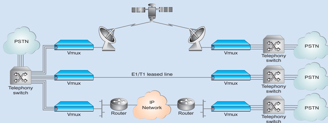
Передача голоса по линиям TDM/IP
