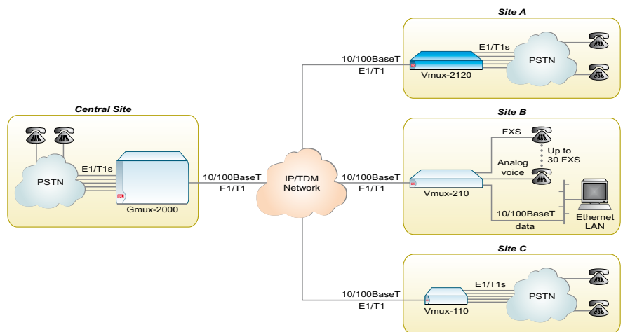
Транспорт трафика голоса по IP/TDM в смешанных топологиях
