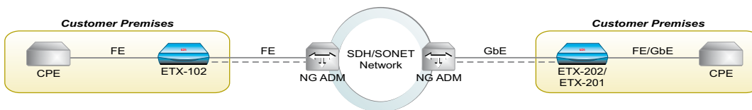
Услуги Ethernet в сетях SDH/SONET нового поколения
