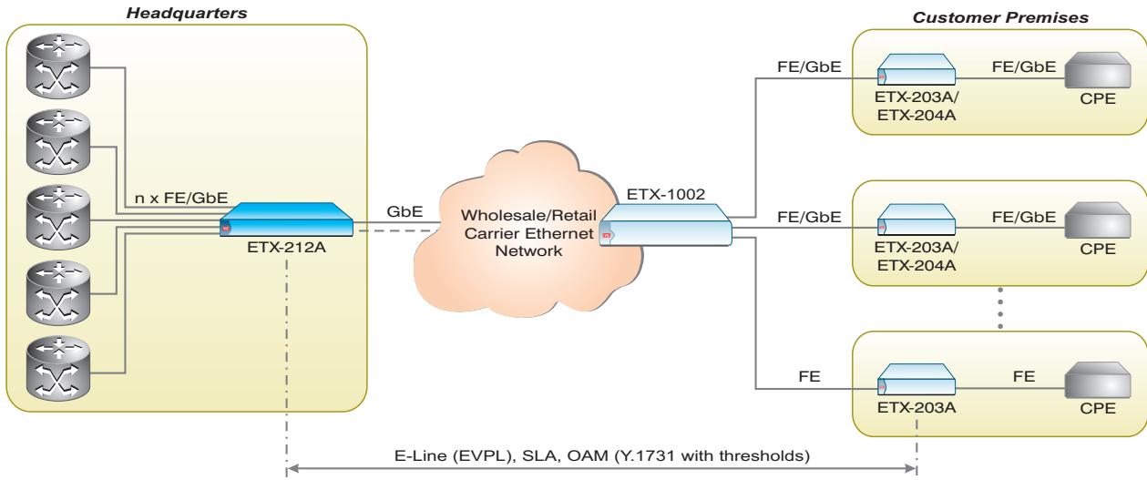
Демаркация услуг Ethernet в пакетных сетях со сквозным обеспечением SLA
