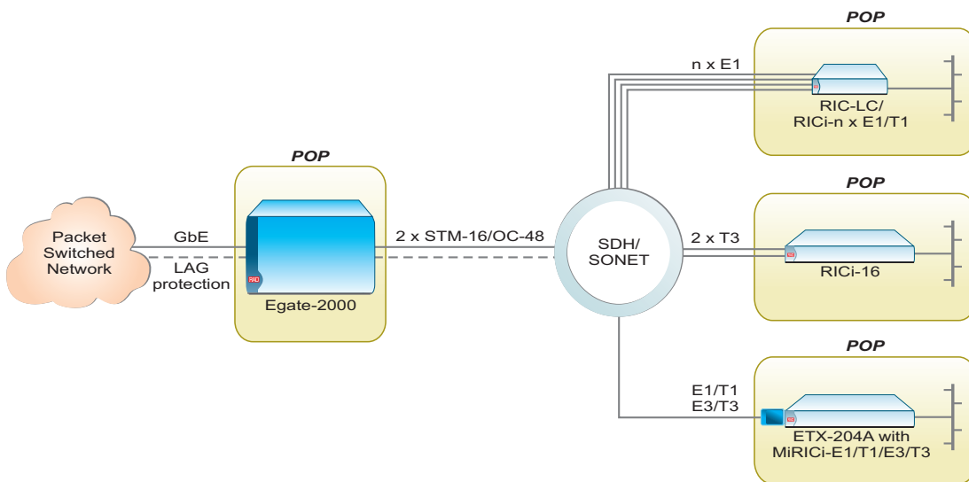
Услуги Ethernet через PDH/SDH/SONET
