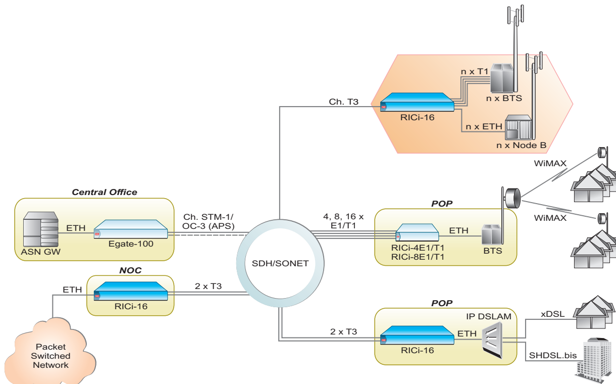
Транспорт услуг по связанным линиям PDH
