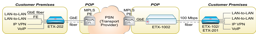
Услуги Ethernet на каждом порту передаются по оптоволокну
