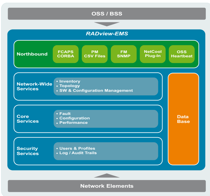
Архитектура RADView-EMS
