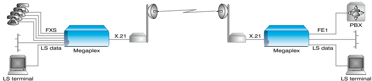
Передача оптимизированного трафика различных услуг по узкополосному каналу с последовательным интерфейсом
