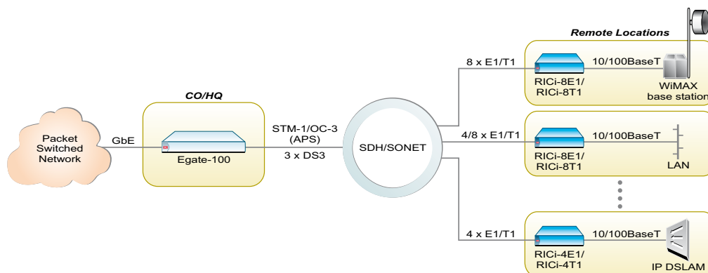
Подключение IP DSLAM и станций WiMAX по каналам n x E1/T1
